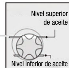
Puerto de comprobación del nivel de aceite del motor
